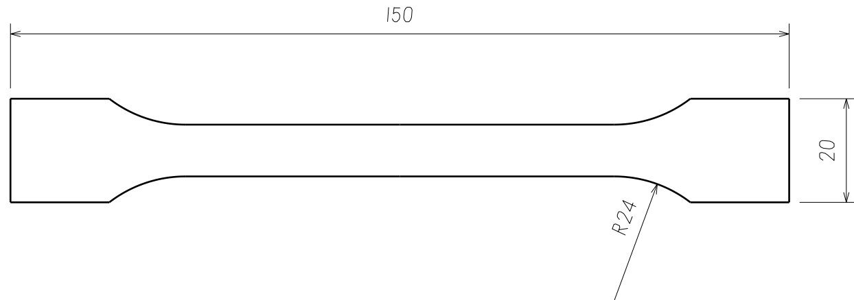
正视图 缩放: 1:1
